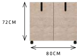
• MÓDULO 2 PUERTAS BATIENTES • - 2 DOOR UNIT -
