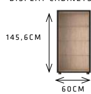
• MÓDULO VITRINA BATIENTE - APERTURA HACIA LA DERECHA • - DISPLAY CABINETS - RIGHT OPENING -
