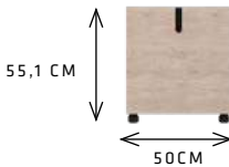
• MÓDULO PUERTA BATIENTE - APERTURA HACIA LA IZQUIERDA • - DOOR UNIT - LEFT OPENING -
